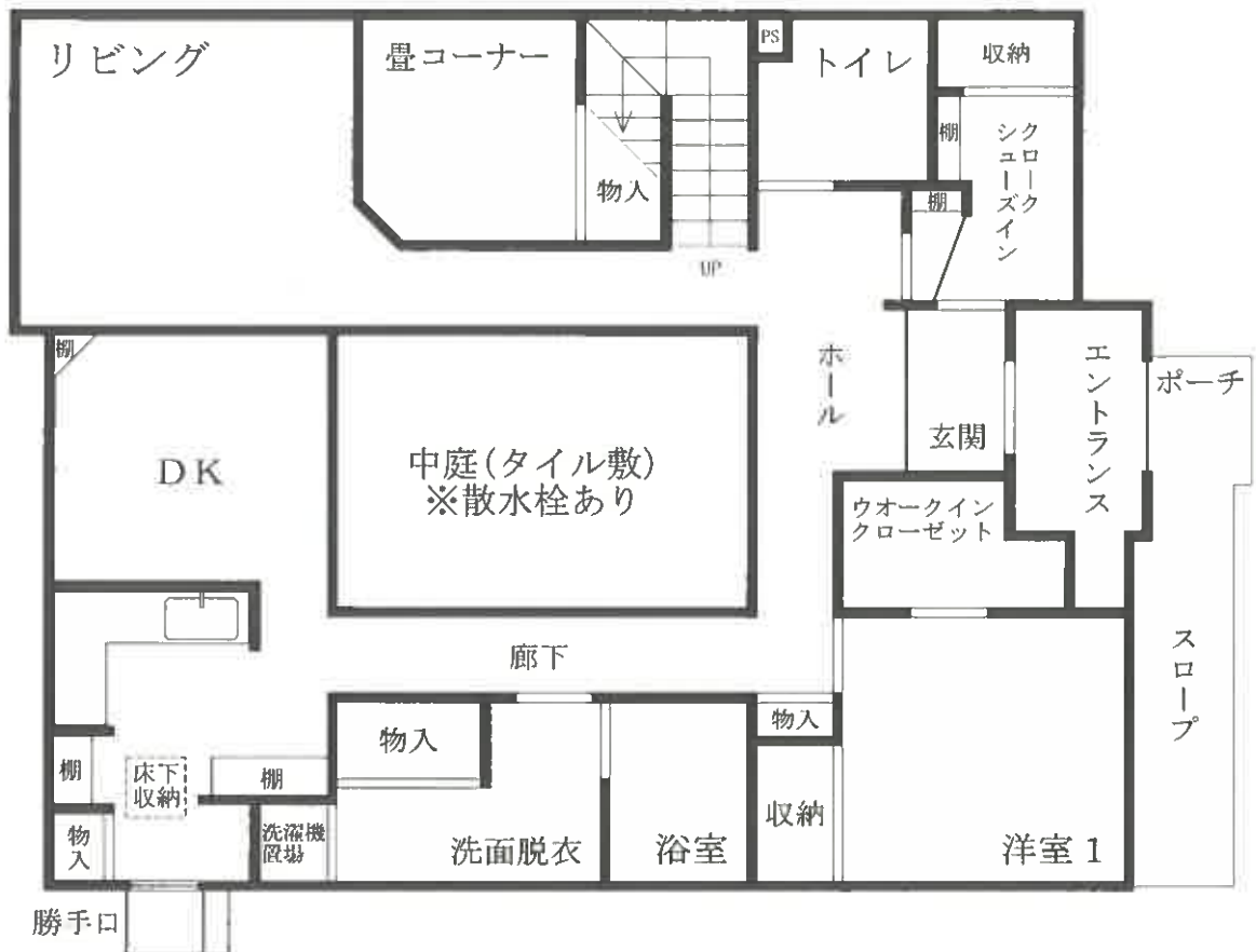
2階 平面図
