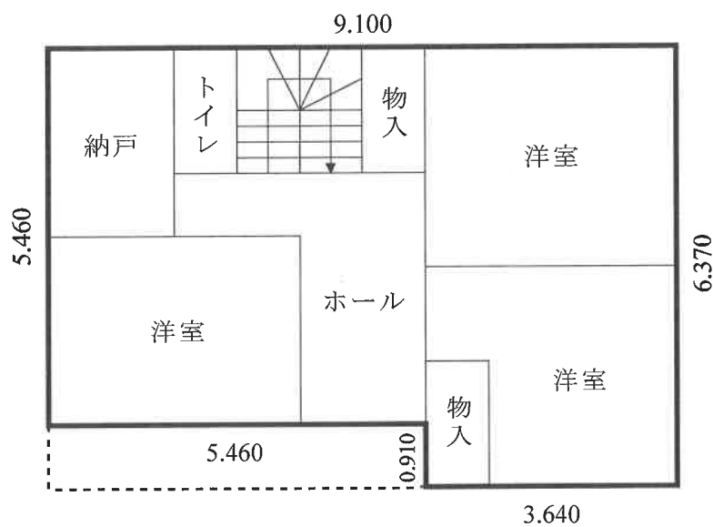
2 階 床面積 5 2.9 9 m 2
