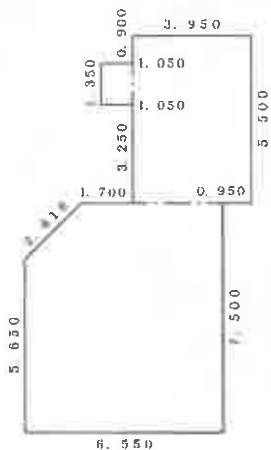
附属建物（符 1）1 階
