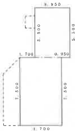
附属建物（符 1）2 階
