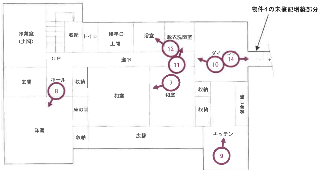
1 階
