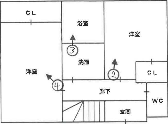
【1階】
