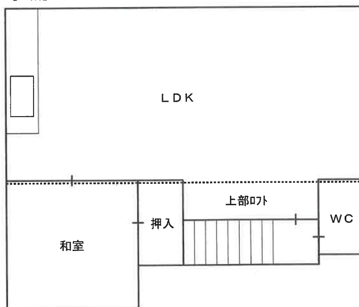
【2階】
