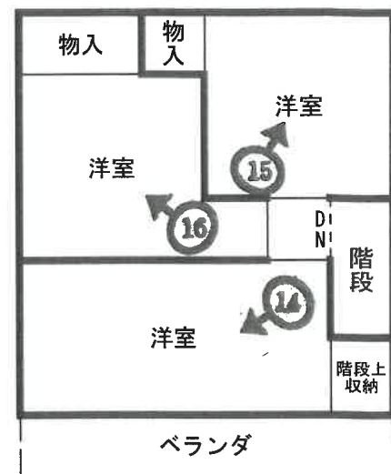
3階平面図
