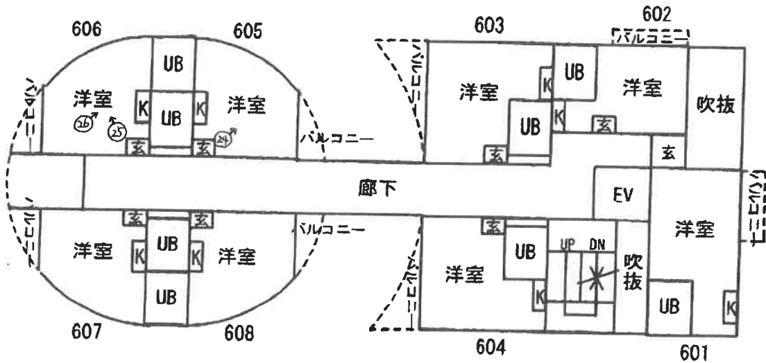
【6階】
