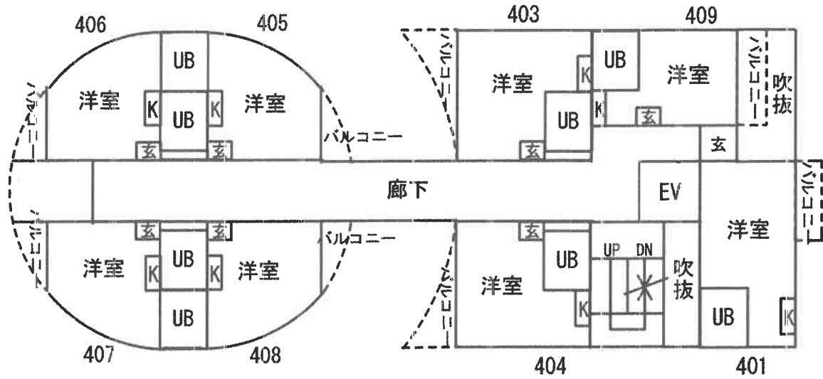
【5階】
