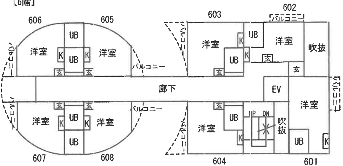
【6階】
