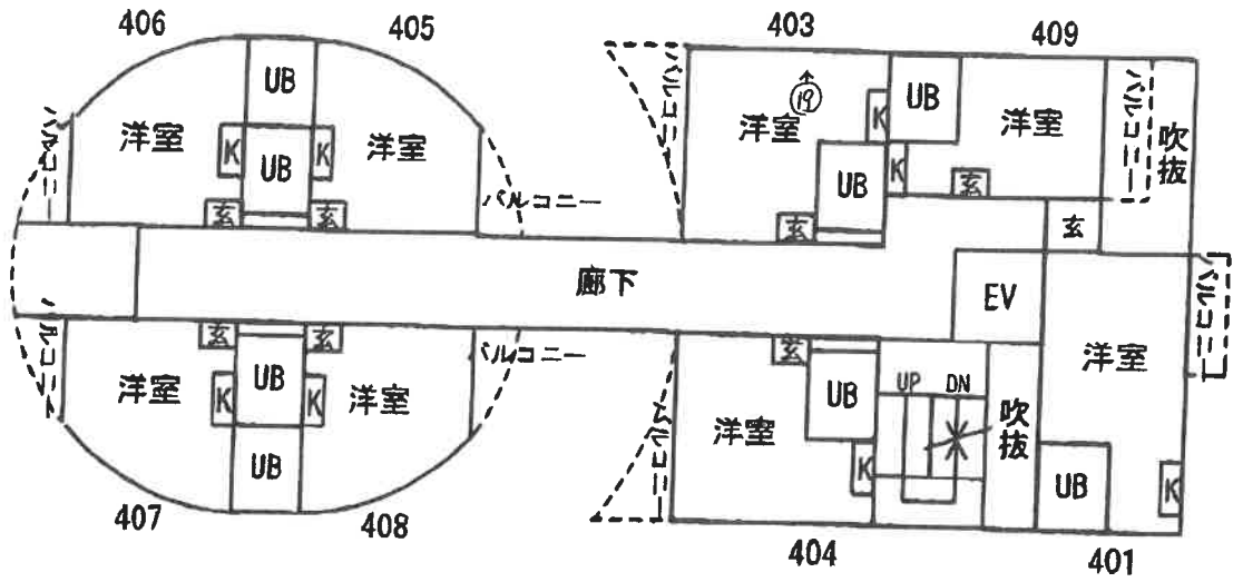
【5階】
