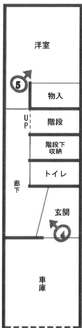
1階平面図
