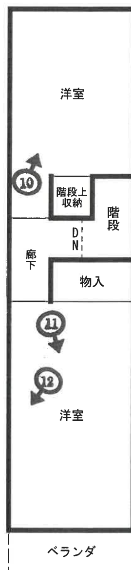
3階平面図
