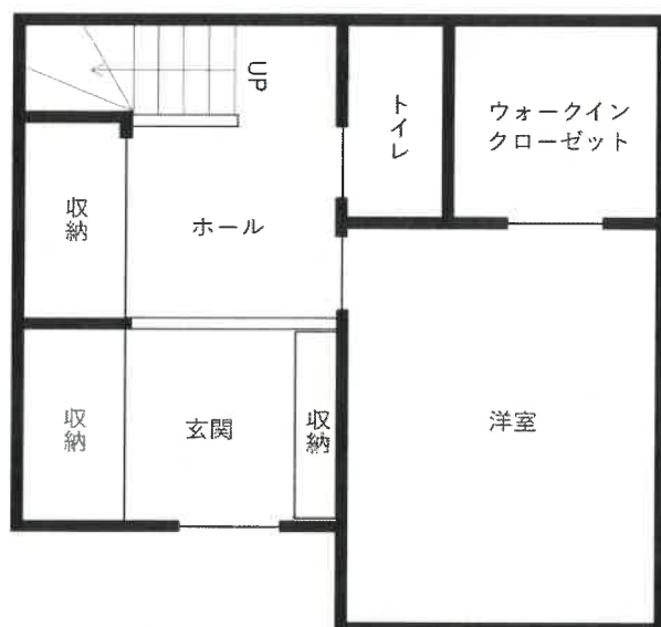
【1階平面図】
