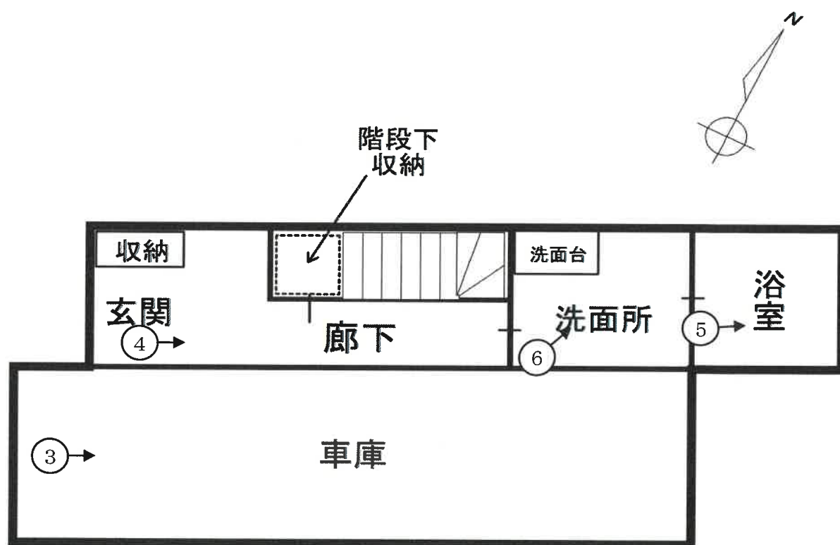
1階
