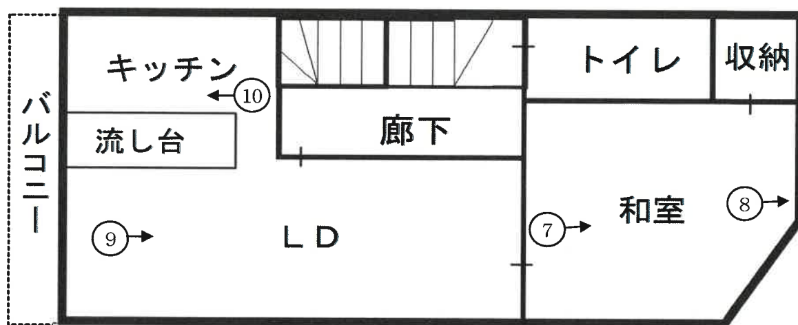
2階
