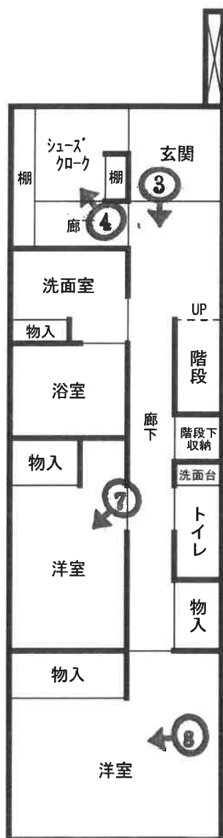
1階平面図
