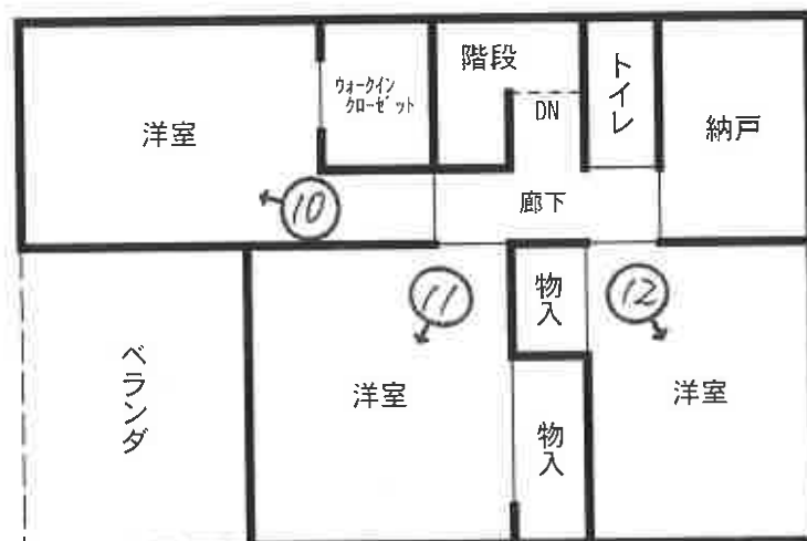
2階平面図
