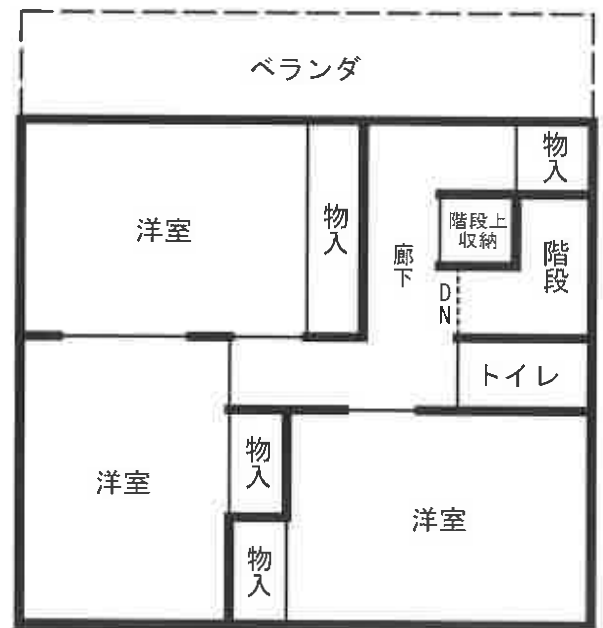
2階平面図
