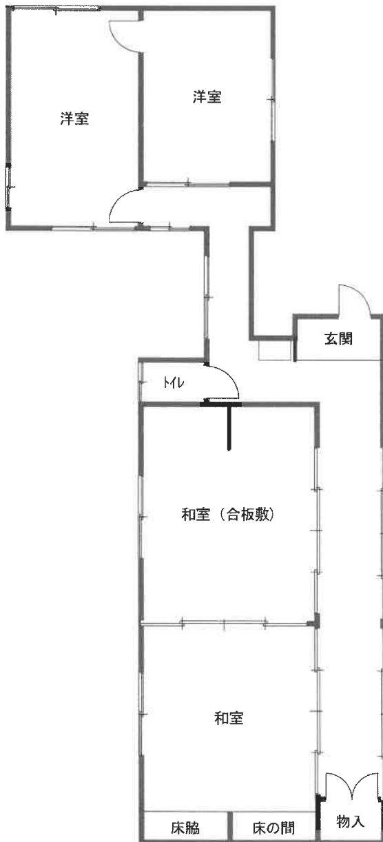
1 階平面図
