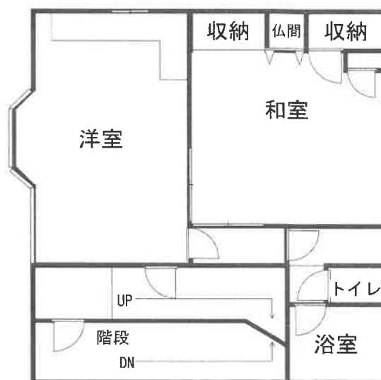
3 階平面図
