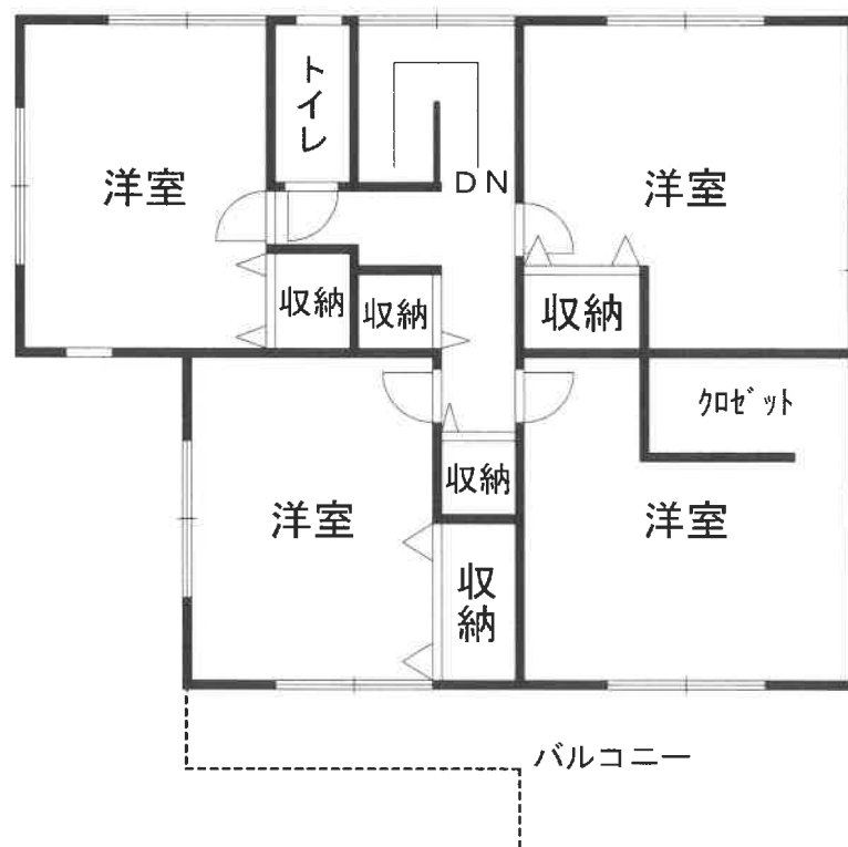
2 階平面図
