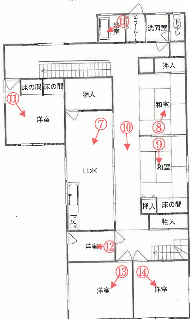
二階平面図
