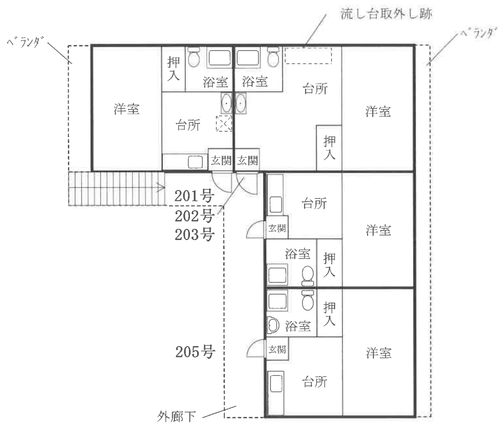
2階
