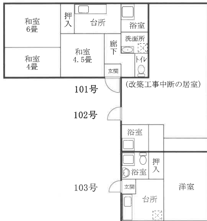
1階
