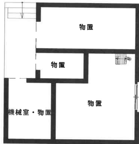
1 階平面図
