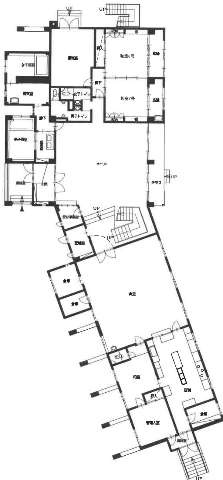
1 階平面図
