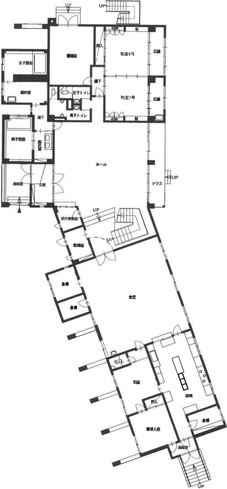
1 階平面図
