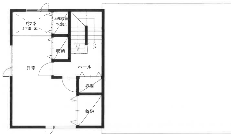
2階平面図 S=1/100
